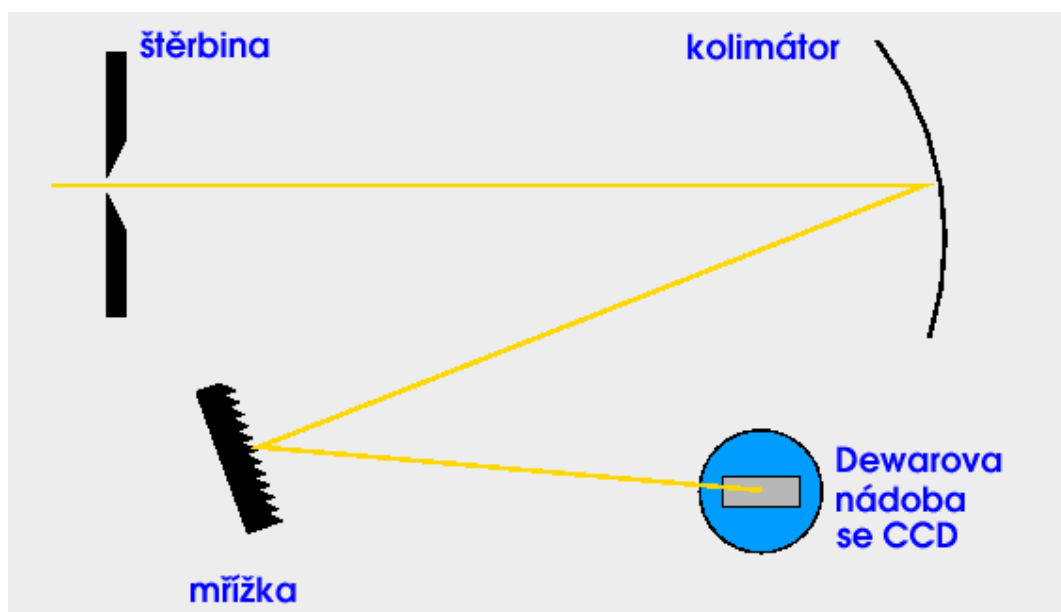
Obr. 3.3: Schéma coudé spektrogratu v Ondřejove [38].
