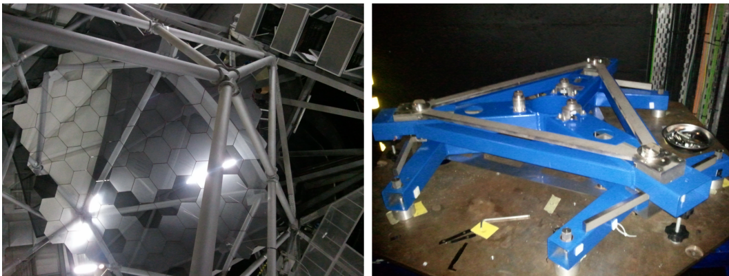
Obrázek 48: Segmentové zrcadlo dalekohledu SALT (South African Large Telescope, Sutherland - vlevo), na kterém je vidět různá kvalita odrazové plochy, vpravo je pak držák jednotlivého segmentu (foto autor).
