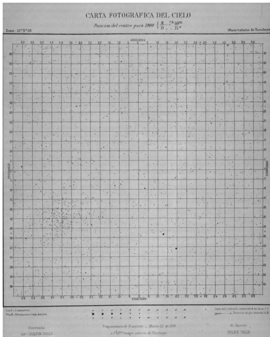
Obrázek 55: Astrometrická fotografie okolí hvězdokupy M46 o rozměrech 2×2 stupně pořízená roku 1909 na observatoře Tacubaya v Mexiku (Gingerich 1984).
