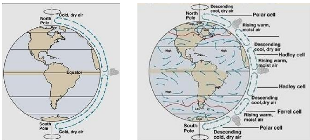
Obrázek 5: Meridiální proudění vzduchu bez a se započtením Coriolisovy síly [E3].
