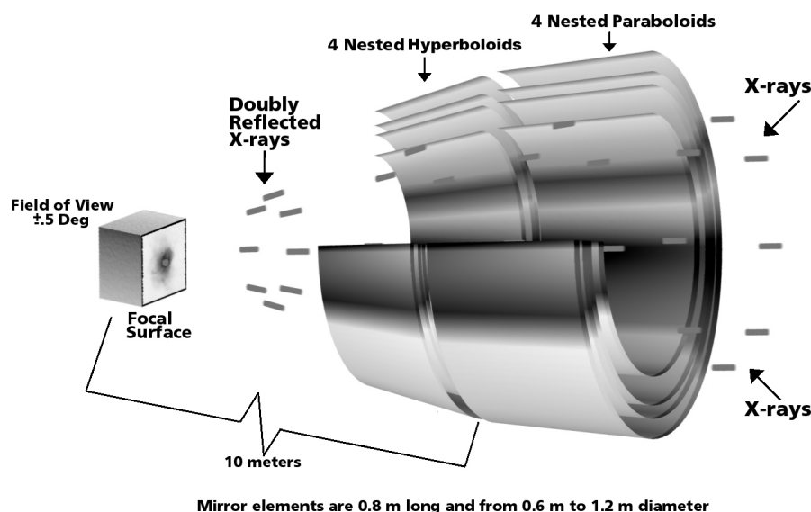
Obrázek 52: Chod paprsků v rentgenovém dalekohledu Chandra [E33].
