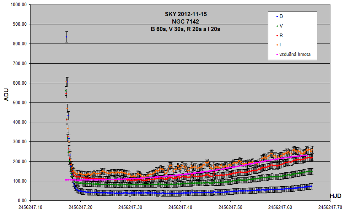
Obrázek 14: Změna jasnosti nebe ve fometrických barvách BVRI během pozorovací noci z 15. na 16. listopadu 2012 na observatoři Suhora v polských Gorcích.
