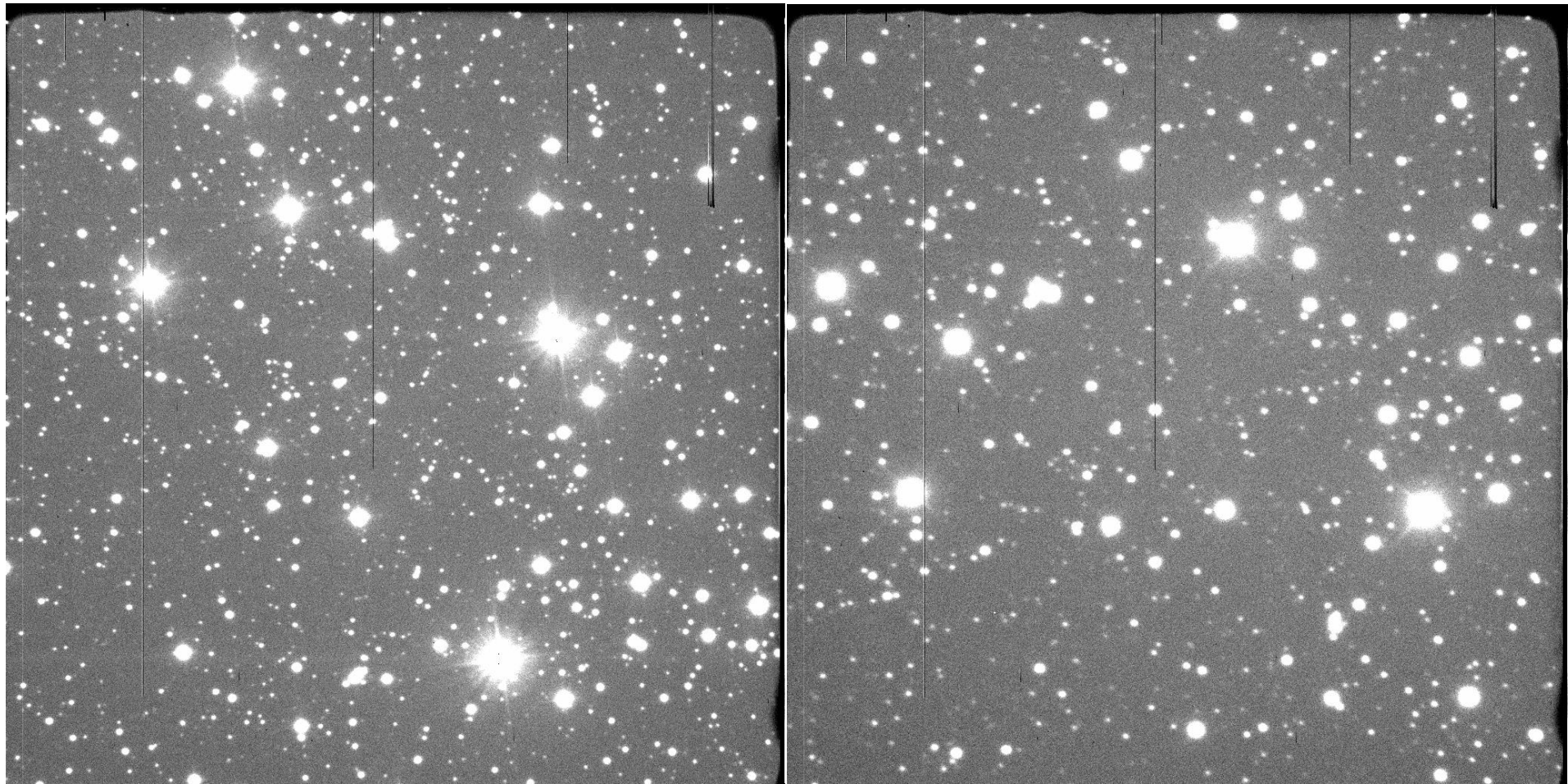
NGC 2910: EFOSC, NTT
