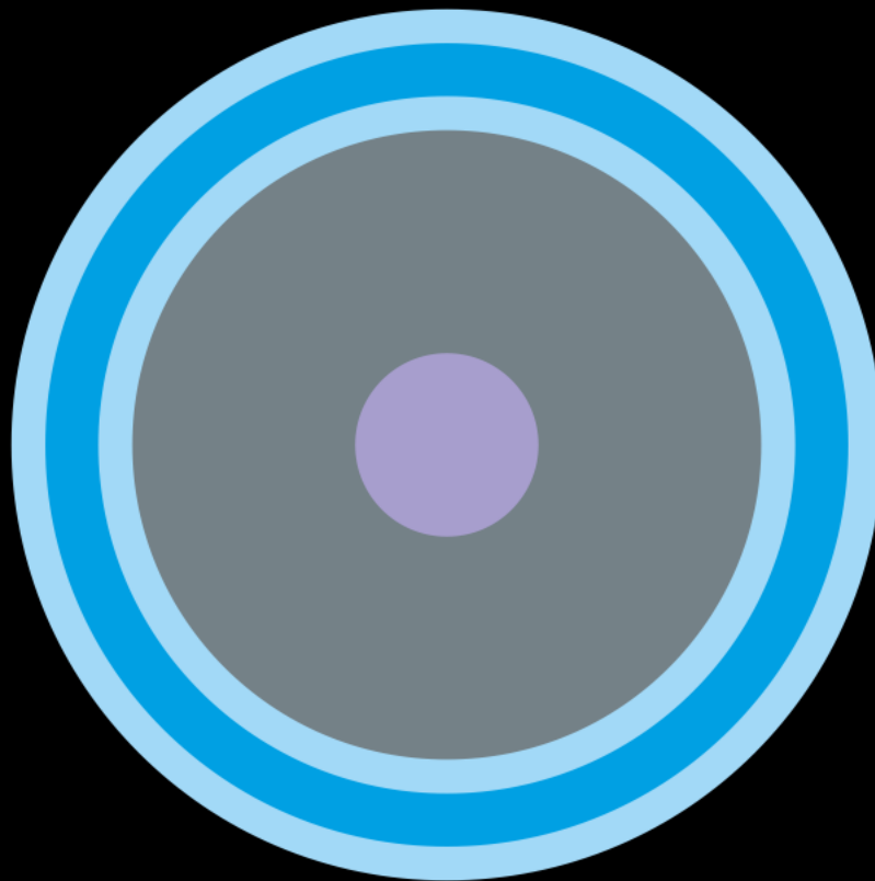
Ganymed
