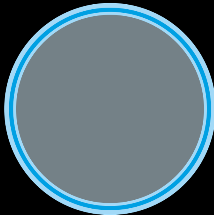
Callisto
